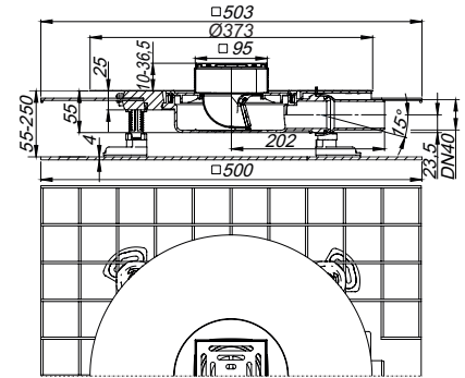
Sumidero insonorizante CeraDrain Pure Plan, 100 x 100 mm
