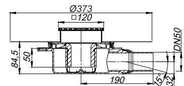
Sumidero DallDrain Pure ABS OM, 120 x 120 mm
