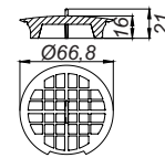
Tamiz fino DalIDrain
