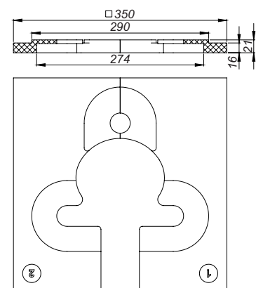
Ayuda de montaje DalIDrain Plan
