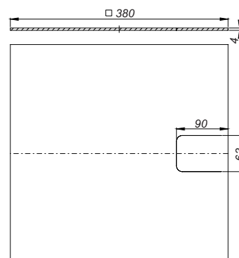
Estera insonorizante DalIDrain
