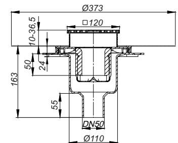
Sumidero DallDrain Pure vertical OM, 120 x 120 mm
