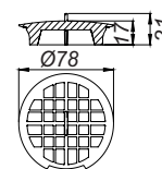
Tamiz fino DalIDrain GM
