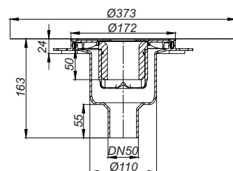
Cazoleta sumidero DallDrain vertical
