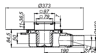
Sumidero DallDrain Individual ABS OM
