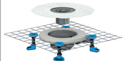
Cazoleta sumidero CeraDrain
