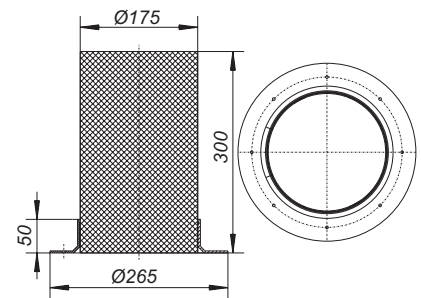
Molde pasa forjado DD 160
