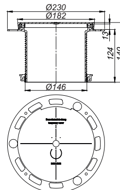
Elemento de elevación DallDrain
