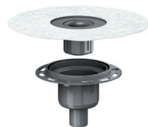
Cazoleta sumidero DallDrain vertical
