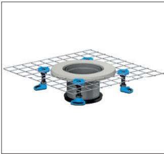
Elemento de elevación CeraDrain Vario Página 63
