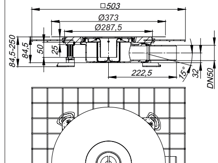
Cazoleta sumidero CeraDrain
