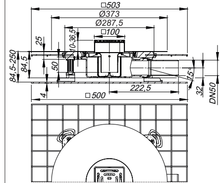
Sumidero insonorizante CeraDrain Select, 100 x 100 mm
