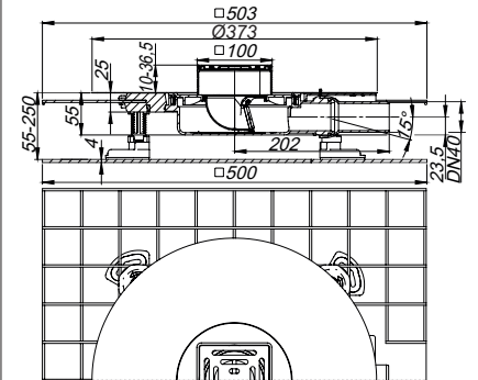
Sumidero insonorizante CeraDrain Select Plan, 100 x 100 mm
