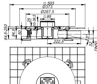
Sumidero CeraDrain Pure 100 x 100 mm
