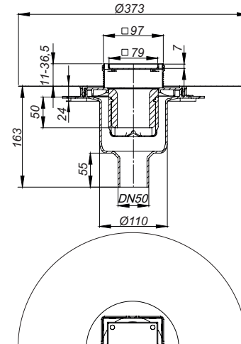
Sumidero DallDrain Individual vertical OM
