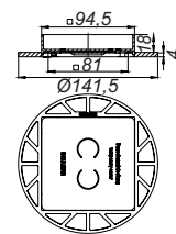
Prolongador DallDrain Individual piedra natural
