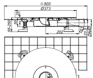
Cazoleta sumidero CeraDrain Plan
