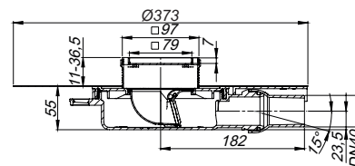
Sumidero DallDrain Individual Plan ABS OM
