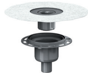
Cazoleta sumidero DallDrain vertical
