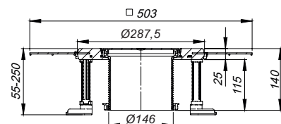
Elemento de elevación CeraDrain Vario
