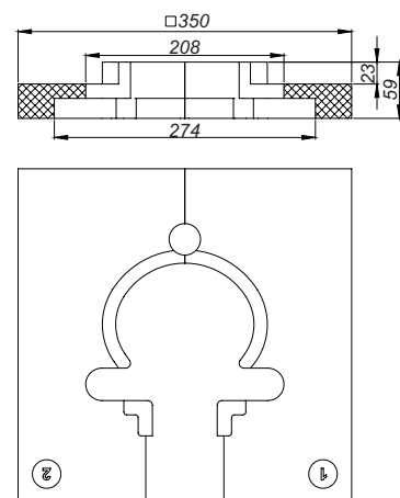
Ayuda de montaje DalIDrain
