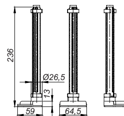
Pies de montaje DallDrain
