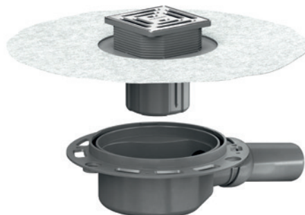
Juego completo ABS OM con cazoleta sumidero DallDrain
