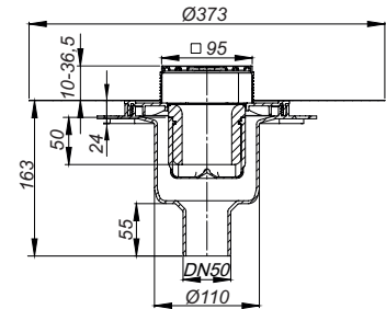
Sumidero DallDrain Pure vertical OM, 100 x 100 mm
