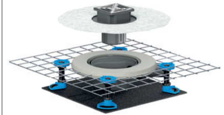
Sumidero insonorizante CeraDrain Select, 100 x 100 mm
