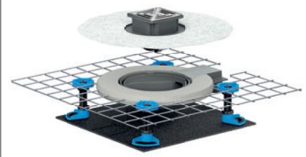
Sumidero insonorizante CeraDrain Select Plan, 100 x 100 mm
