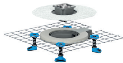
Sumidero CeraDrain Pure Plan, 100 x 100 mm
