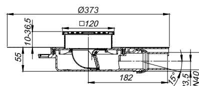
Sumidero DalIDrain Pure Plan ABS OM, 120 x 120 mm
