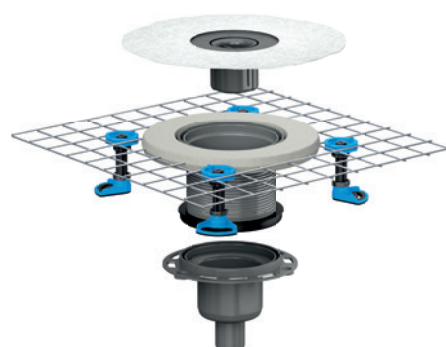
DallDrain vertical + CeraDrain Vario
