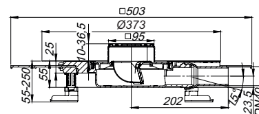
Sumidero CeraDrain Pure Plan, 100 x 100 mm
