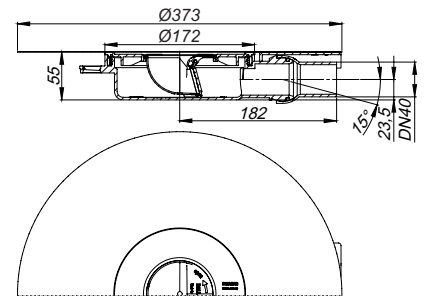
Cazoleta sumidero DallDrain Plan ABS
