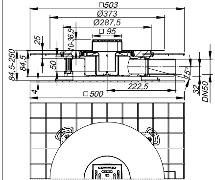
Sumidero insonorizante CeraDrain Pure, 100 x 100 mm
