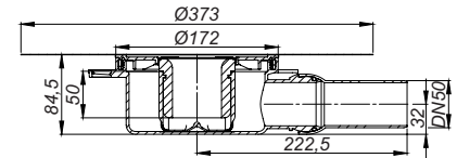
Cazoleta sumidero DalIDrain ABS
