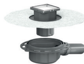
Sumidero DallDrain Individual ABS OM
